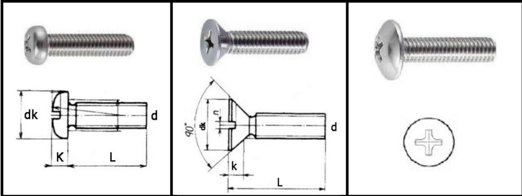
สกรูมิลซบขาว หัวกลม JP หัวเตเปอร์ JF หัวกะทะ JT
